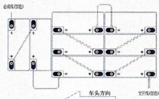
电池连接示意图
